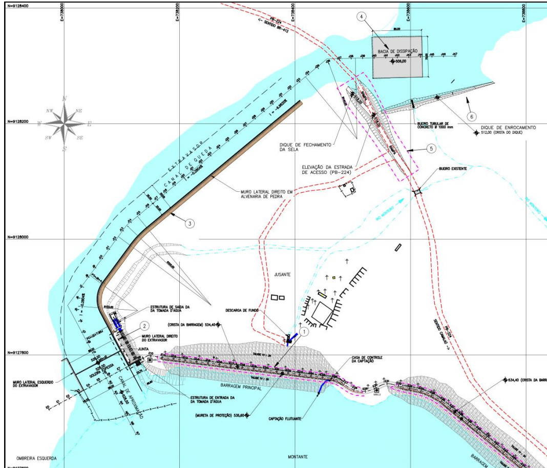
FIGURA 4.2 - ELEVAÇÃO DA CRISTA DAS BARRAGENS PRINCIPAL E AUXILIAR E EXECUÇÃO DE MURO LATERAL DIREITO DO EXTRAVASOR EM ALVENARIA DE PEDRA
