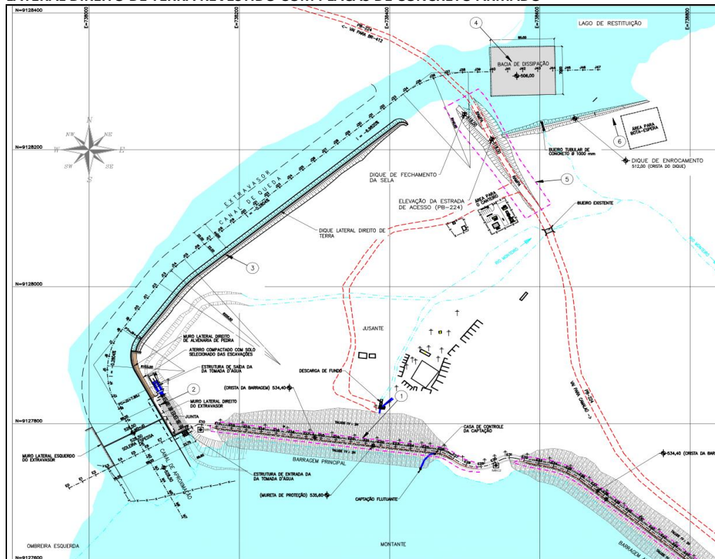
FIGURA 4.4 - ELEVÇÃO DA CRISTA DAS BARRAGENS PRINCIPAL E AUXILIAR E EXECUÇÃO DE UM DIQUE LATERAL DIREITO DE TERRA REVESTIDO COM PLACAS DE CONCRETO ARMADO
