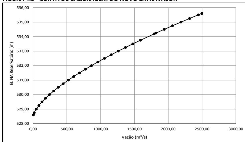
FIGURA 4.5 - CURVA DE CALIBRAGEM DO NOVO EXTRAVASOR
