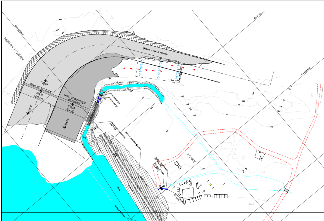
FIGURA 4.1 - AMPLIAÇÃO DO EXTRAVASOR
