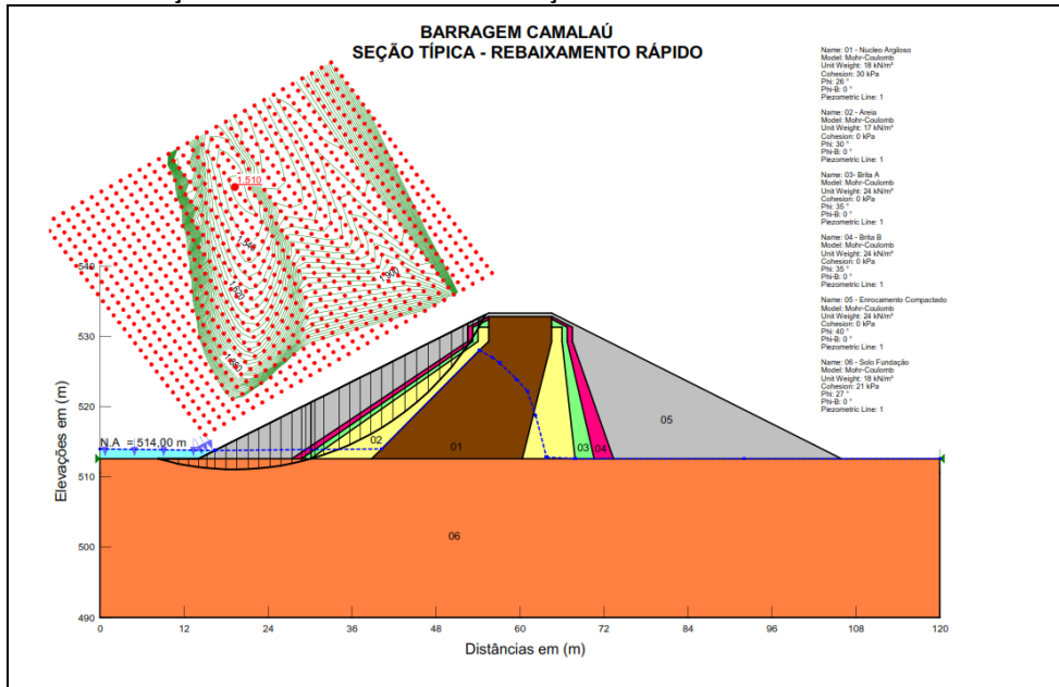
FIGURA 4.9 - SEÇÕES CRÍTICAS ANALISADAS - MACIÇO EXISTENTE - REBAIXAMENTO RÁPIDO
