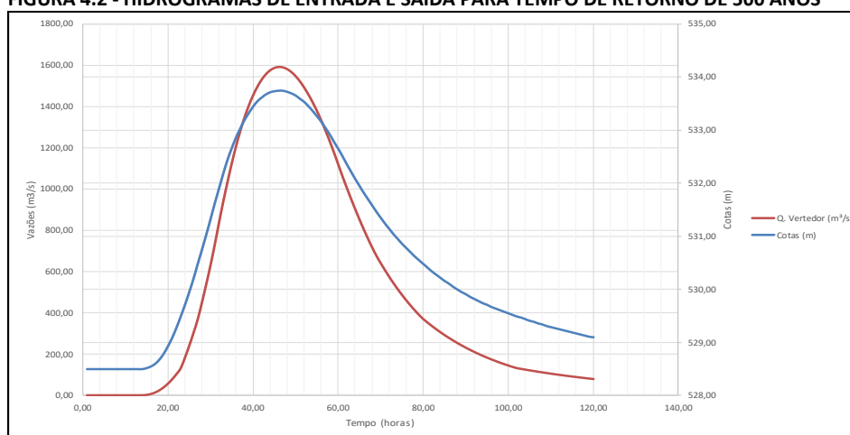
FIGURA 4.2 - HIDROGRAMAS DE ENTRADA E SAÍDA PARA TEMPO DE RETORNO DE 500 ANOS
